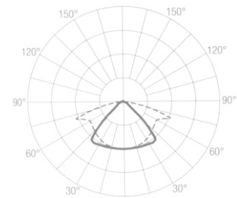
Curva de distribución de la luz 90°
