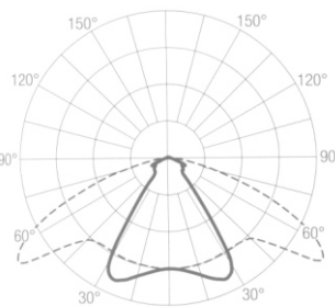
Curva de distribución de la luz 60°
