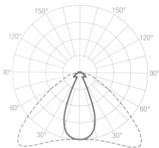
Curva de distribución de la luz 30°
